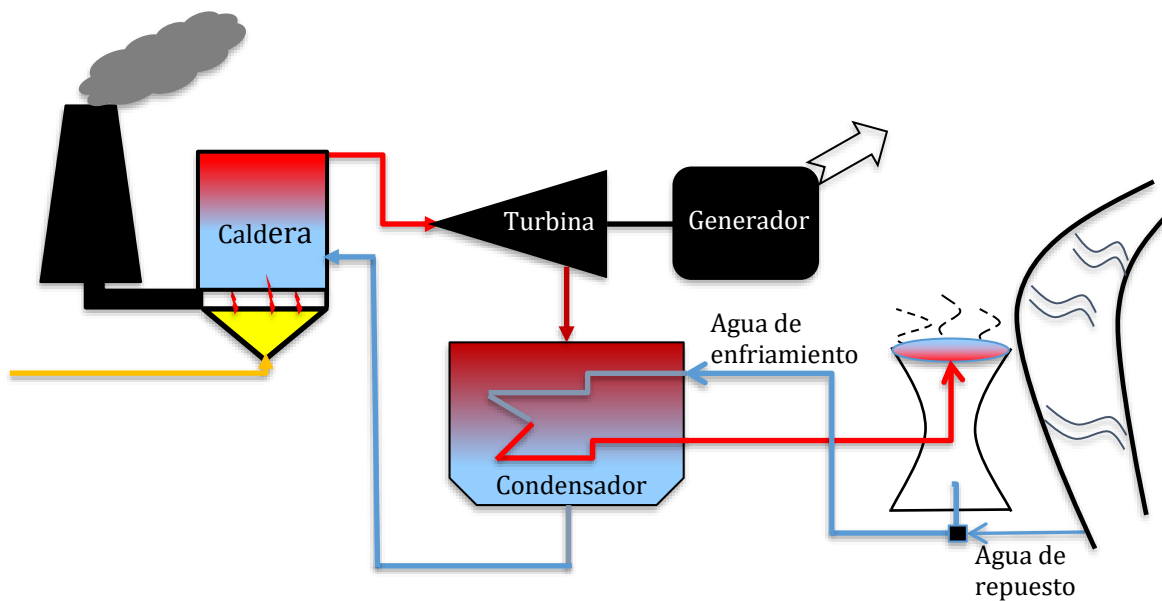
Figura 3.11. Sistema de enfriamiento empleado por una central termoeléctrica. La torre de enfriamiento evita la contaminación térmica del río, pero éste debe suministrar agua de reposición.
