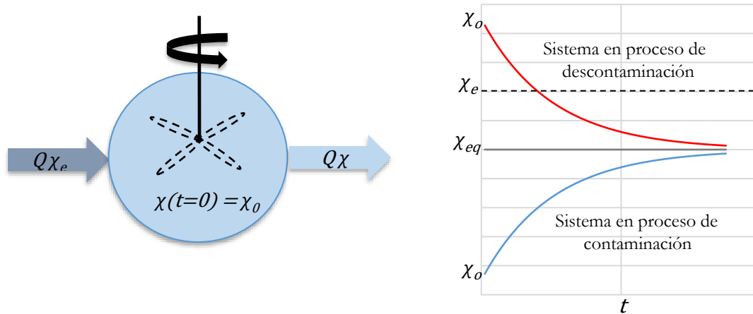
Figura 3.6. Evolución de una sustancia reactiva , siguiendo una reacción de orden 1 con degradación, dentro de un sistema bien mezclado con una entrada y una salida de material. Al final del proceso, independientemente del valor de la concentración inicial, el sistema se estabiliza adquiriendo el valor de la concentración de equilibrio; esta concentración invariablemente será menor que la concentración de entrada.
