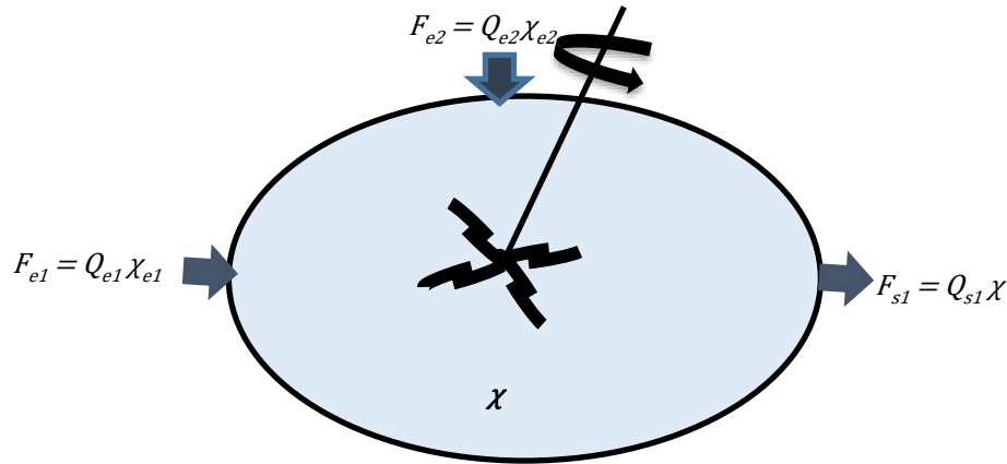
Figura 3.3. Un sistema constituido por un lago bien mezclado. El mezclado provoca una concentración homogénea en todo el sistema que incluye el sitio de salida del material.
